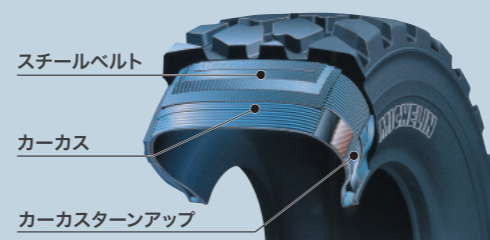
※ローダー用タイヤ断面図
